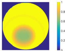
(d) D-bar [24]
