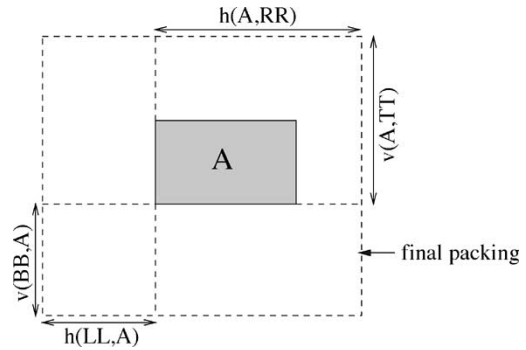
Fig. 2. Notations h(LL, A) , h(A, RR) , v(BB, A) and v(A, TT) .
