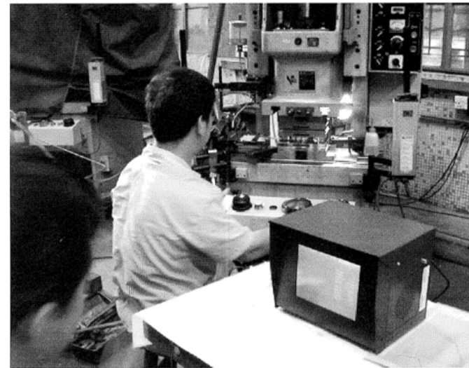
金屬沖壓在線監控與診斷系統的試用型產品
