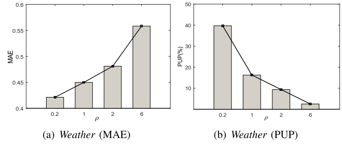
Fig. 6. Evaluation on parameter \rho .
