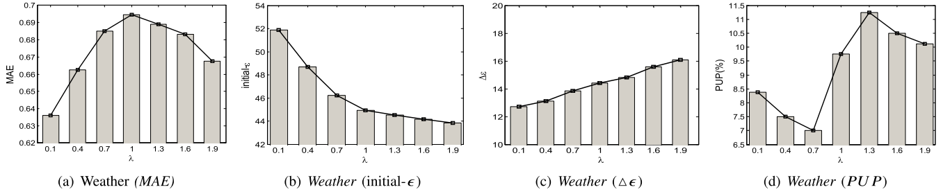
Fig. 4. Evaluation on parameter \lambda .
