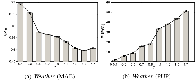
Fig. 7. Evaluation on parameter \gamma .
