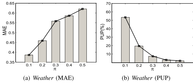
Fig. 5. Evaluation on parameter \pi .
