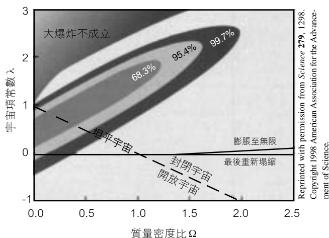
根據最新測量結果所推斷得 \lambda 與 \rho 值的分布：圖中百分率指分布的預期值。宇宙斥力與 \lambda 成比例；質量密度比 \Omega = \rho / \rho_c ( \rho_c 為臨界密度， \rho_c 及 \Omega 的意義見本刊26，86，1994年12月號)。
