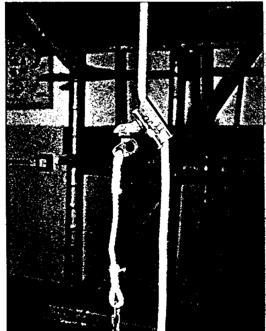
連接安全帶的懸掛繩和獨立救生繩的防墮器。
