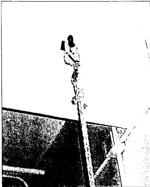
應以有眼螺栓作為懸掛獨立救生繩的固定錨點。
