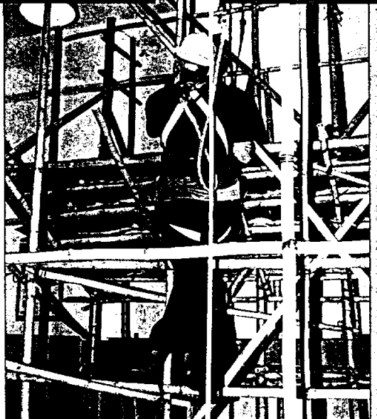
安全帶必須繫緊於可承受不少於5000牛頓拉力(約510公斤拉力)的固定錨點或獨立救生繩上。
