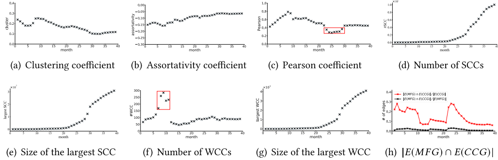
Fig. 8. Trend of MFG.
