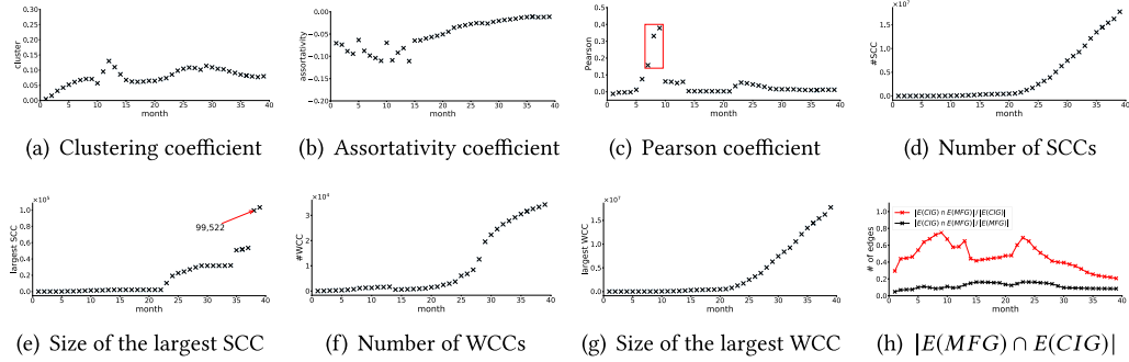
Fig. 13. Trend of CIG.
